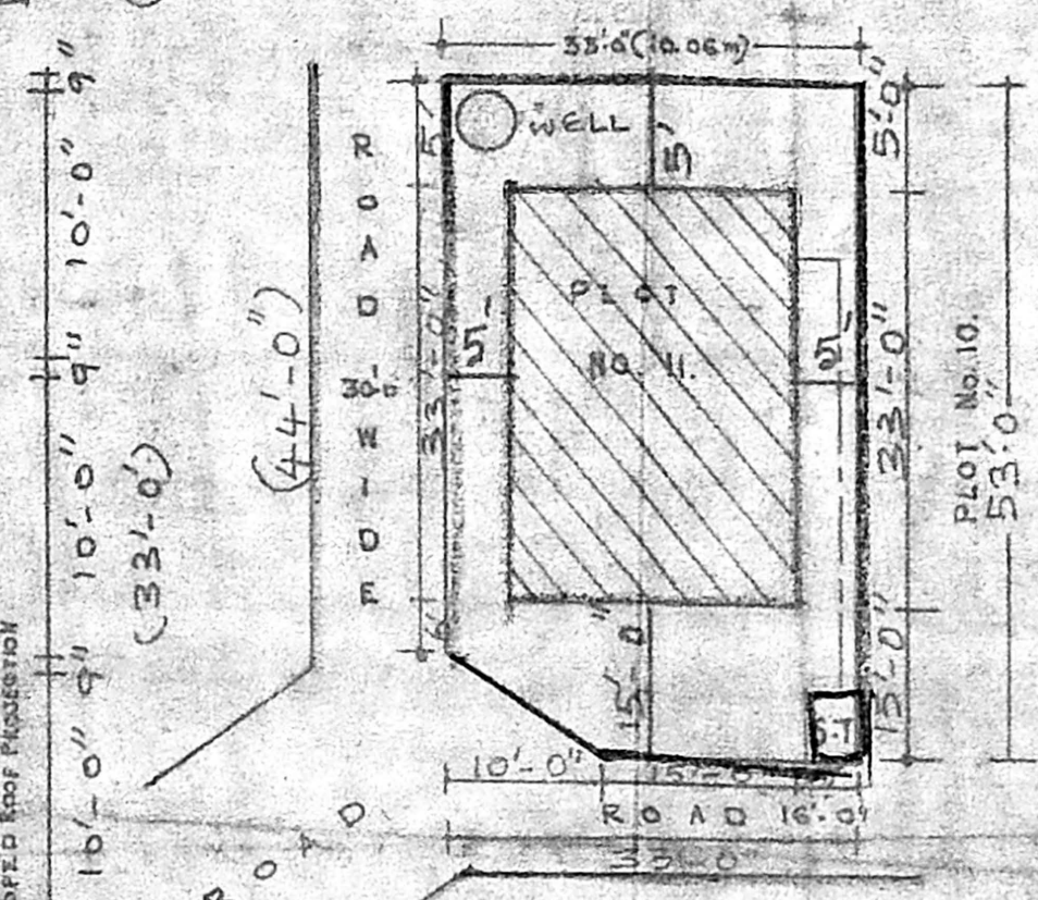
SITE PLAN SCALE: 1CM 5M.
